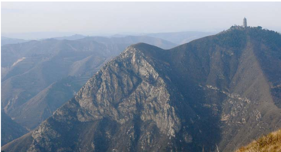
圖 06 此是谷口西山—黃山的東面，在輞谷內，石質顯豁，坡度深峭，不適人居。谷口外西北面的鞍部，土厚坡緩，才適合建築，後文另有照片。拍攝於七盤嶺第二重稜線西端 34^{\circ}5'16.80''\text{N} ， 109^{\circ}20'28.79''\text{E} 處，角度約 270^{\circ}
